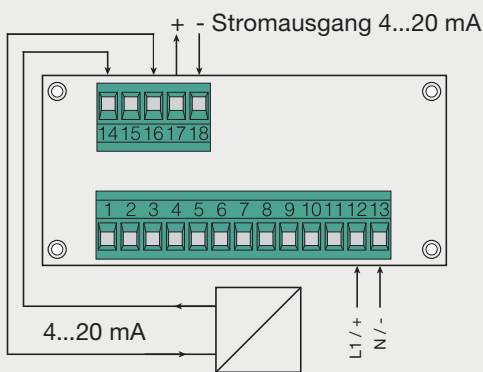
Abb. 3: Elektrischer Anschluss | 0/4...20 mA
