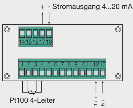
Abb. 2: Elektrischer Anschluss | Pt100 4-Leiter
