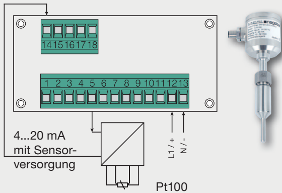
Abb. 1: Elektrischer Anschluss | Zweileitermessumformer
