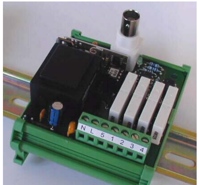
Funkfernsteuer-Empfänger EFB-EK4-UM72-BNC
